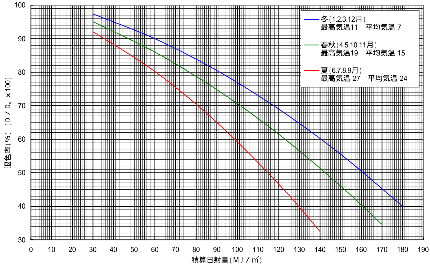
オブリーフ退色曲線(検量線) 「Y-1W」 日射量 (千葉市実測値)
